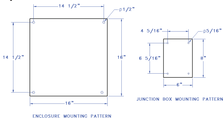
Diagram 9A. Mounting detail.
